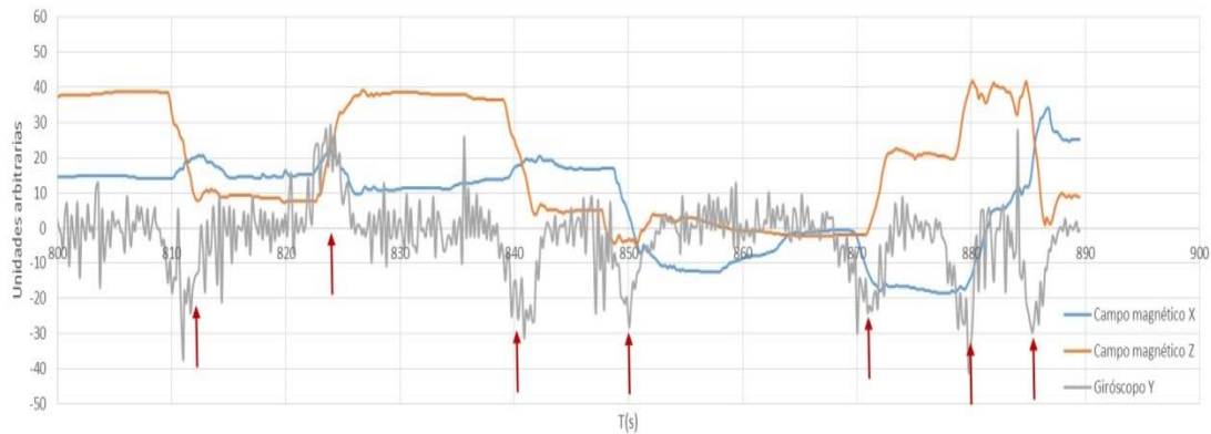
Figura 4. Componentes horizontales X , Z del campo magnético y componente vertical Y del giróscopo. En rojo flechas que señalan los puntos donde el vehículo gira.
