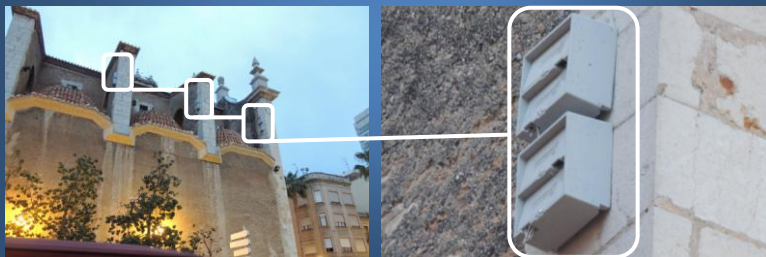
Solució adoptada en la restauració de l'església de Sant Bartomeu, a Benicarló
